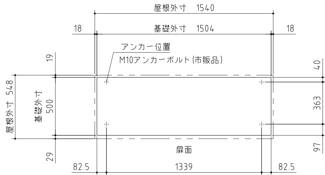
ベタ基礎図
